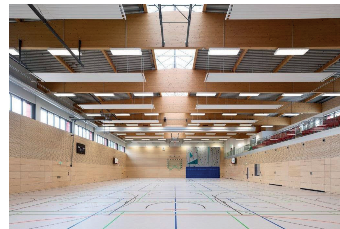
Polizeiakademie Hann. Münden, Neubau Sporthalle
